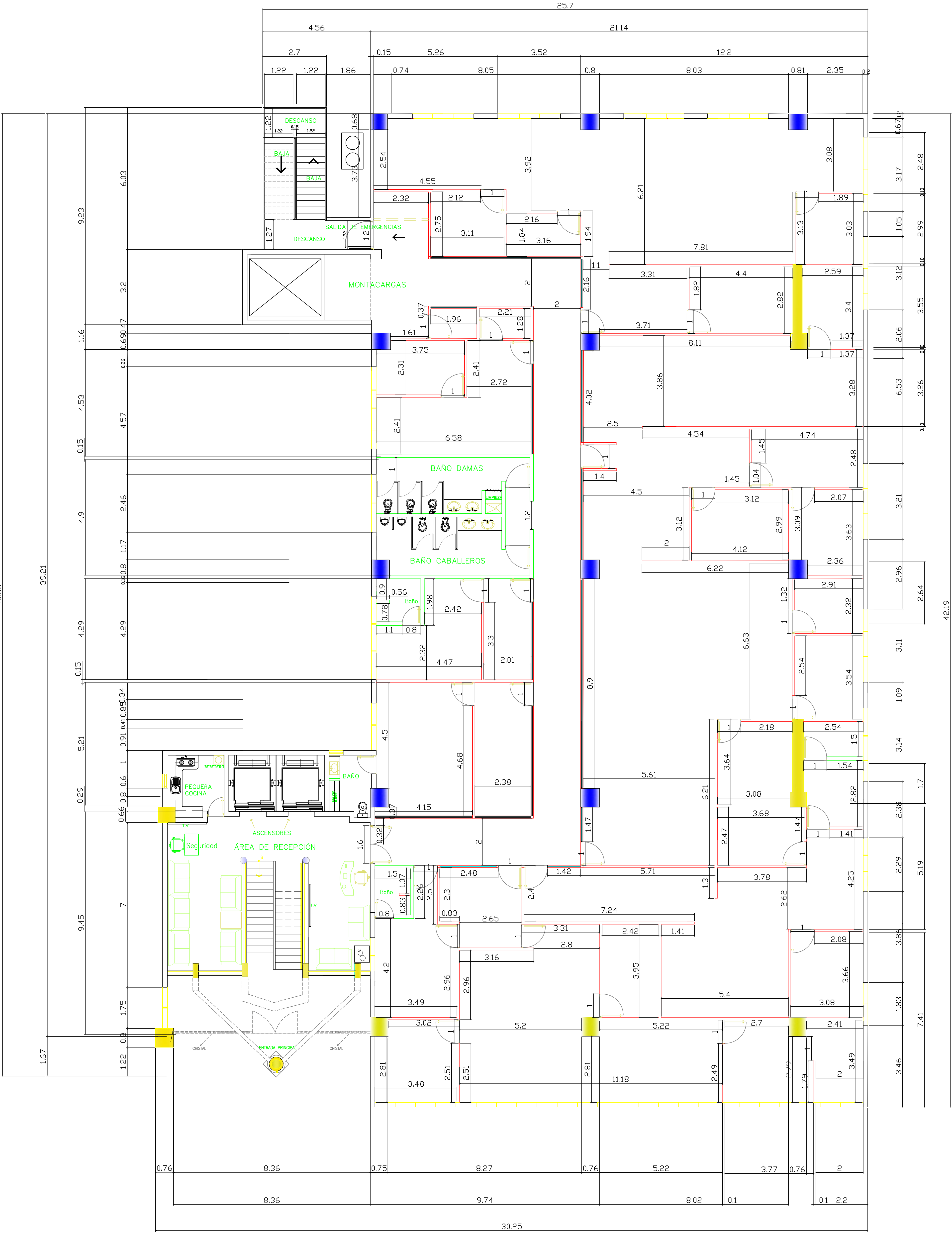
PLANTA DIMENSIONADA - TORRE INABIE (NIVEL 2)
