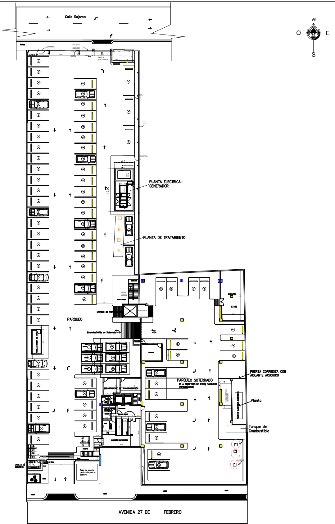
PLANTA PARQUEOS - TORRE INABIE
