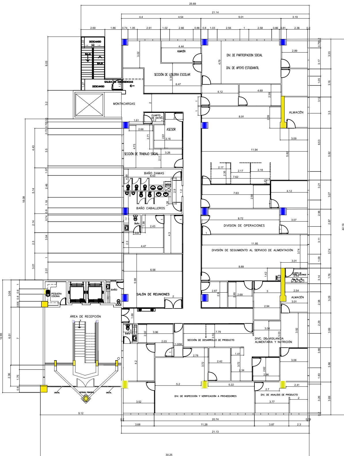
PLANTA DIMENSIONADA- TORRE INABIE (NIVEL 2)
