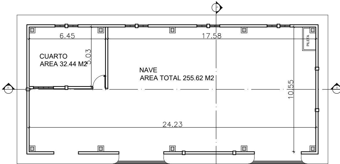
1 PLANTA ARQUITECTONICA NAVE A-3 ESC. 1:75
